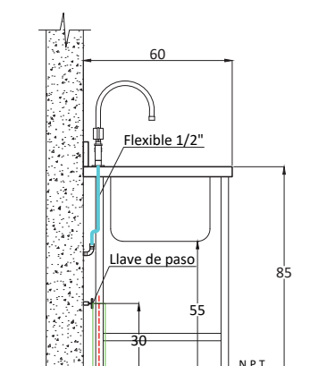
ELEVACIÓN LATERAL
