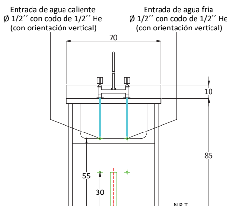
ELEVACIÓN FRONTAL
